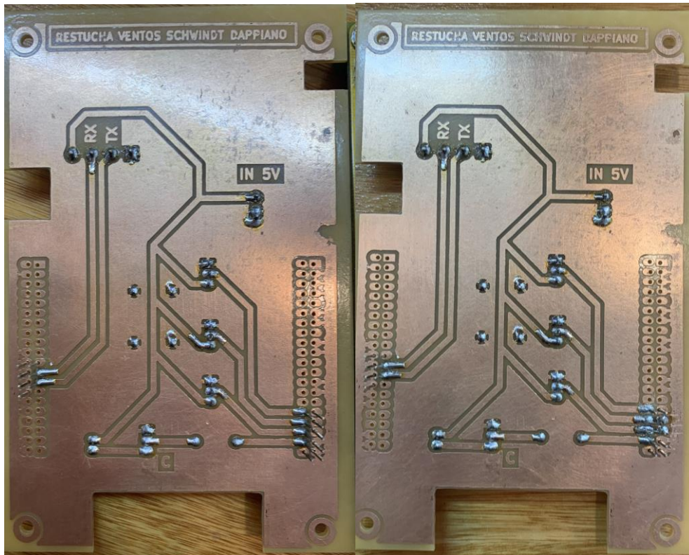
4.2.2.c PCB antes de corrección de pines.
