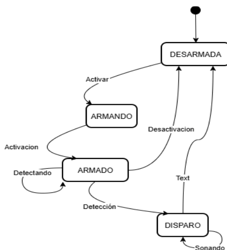
Figura 5.4: Diagrama de Moore sencillo como FSM
